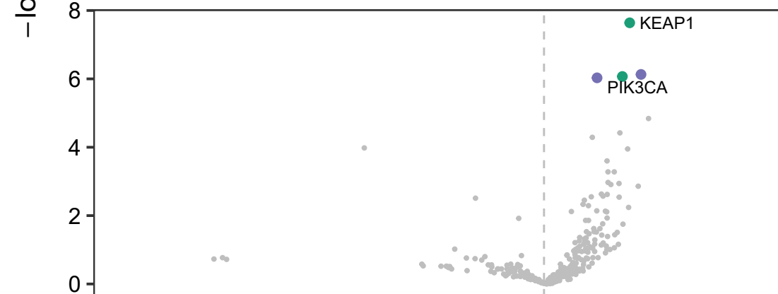
KRAS Codon 13
