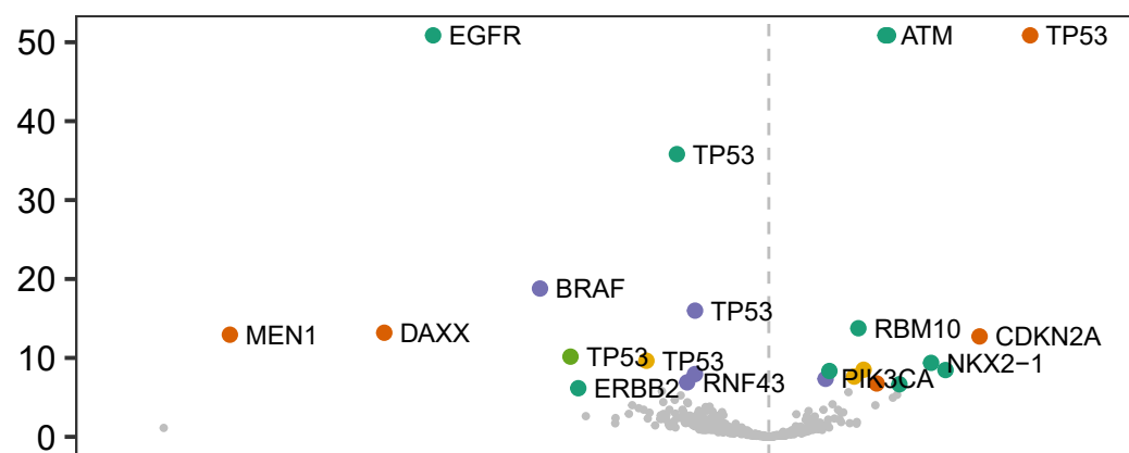
KRAS Codon 12
