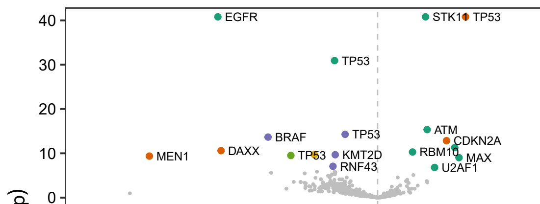
KRAS Codon 12
