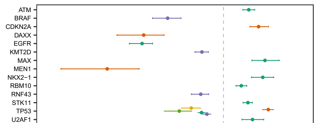
KRAS Codon 12
