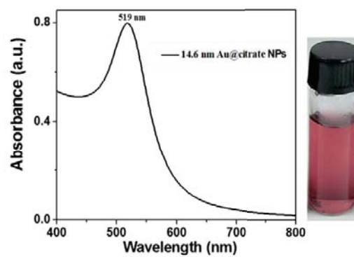
C: UV-vis
