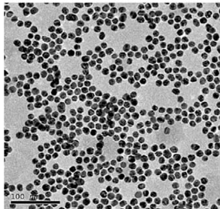
A: TEM
