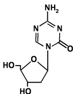
Decitabine
