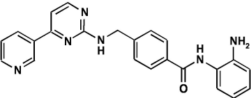
MGCD0103
